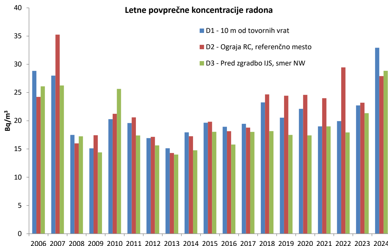
Graf 5: Povprečne letne koncentracije radona v okolici objekta CSRAO.
