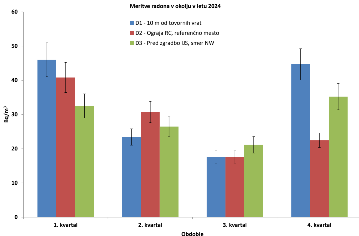
Graf 4: Povprečna koncentracija radona v okolici objekta CSRAO (po kvartalih)
