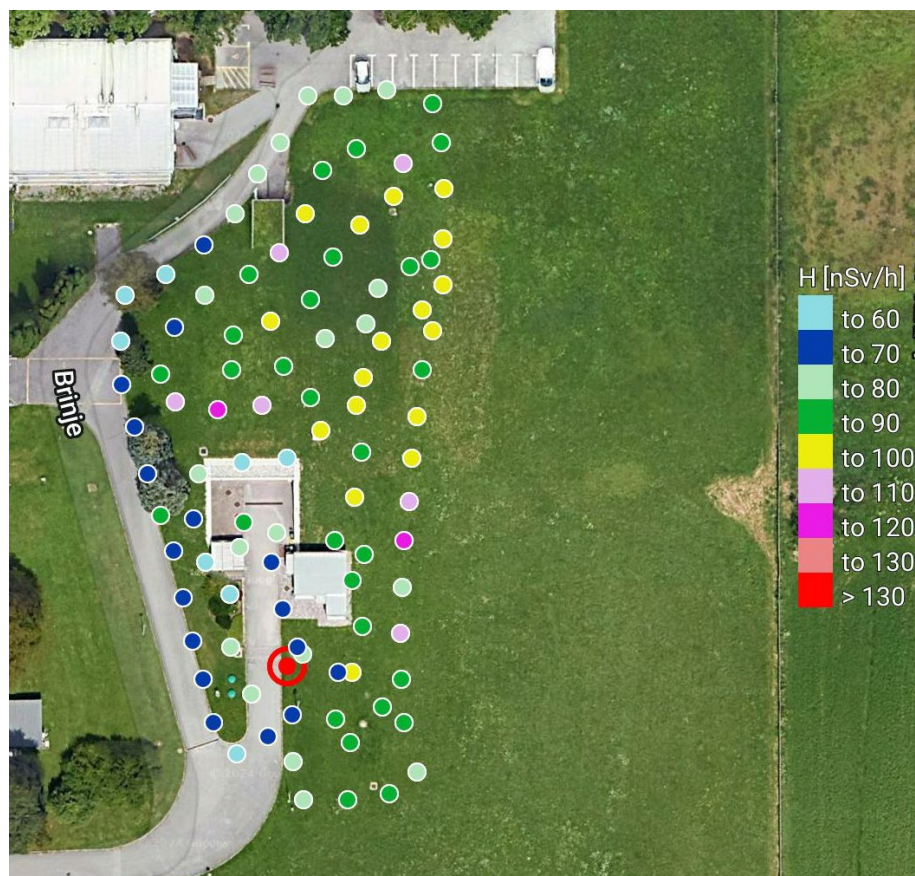
Slika 2: Rezultati meritev hitrosti doze H^*(10)[nSv/h] sevanja gama v ožji in širši okolici objekta CSRAO, predstavljeni s programsko opremo Route Monitoring (julij 2024)
