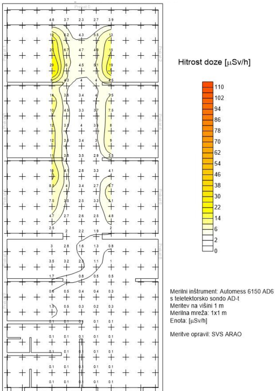
Slika 3: Izmerjene vrednosti hitrosti doze gama ( \mu\text{Sv/h} ) dne 8. 8. 2024 na transportni poti s prenosnim merilnikom v CSRAO.
