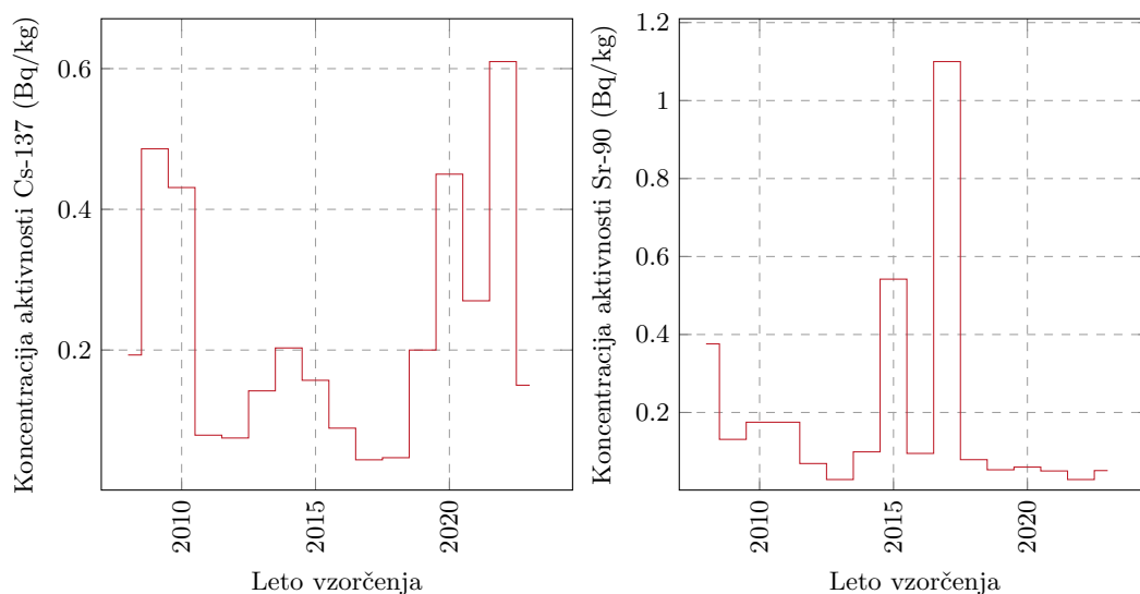
Slika 5.9 | Povprečne letne koncentracije aktivnosti Cs-137 in Sr-90 v živilih živalskega izvora od leta 2008 dalje (povprečje vseh vzetih vzorcev razen medu in divjačine).
