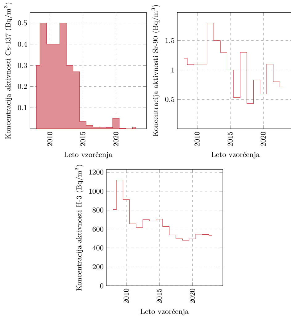
Slika 5.2 | Povprečne letne koncentracije aktivnosti Cs-137, Sr-90 in H-3 v pitni vodi od leta 2009 dalje (povprečje vseh vzetih vzorcev).
