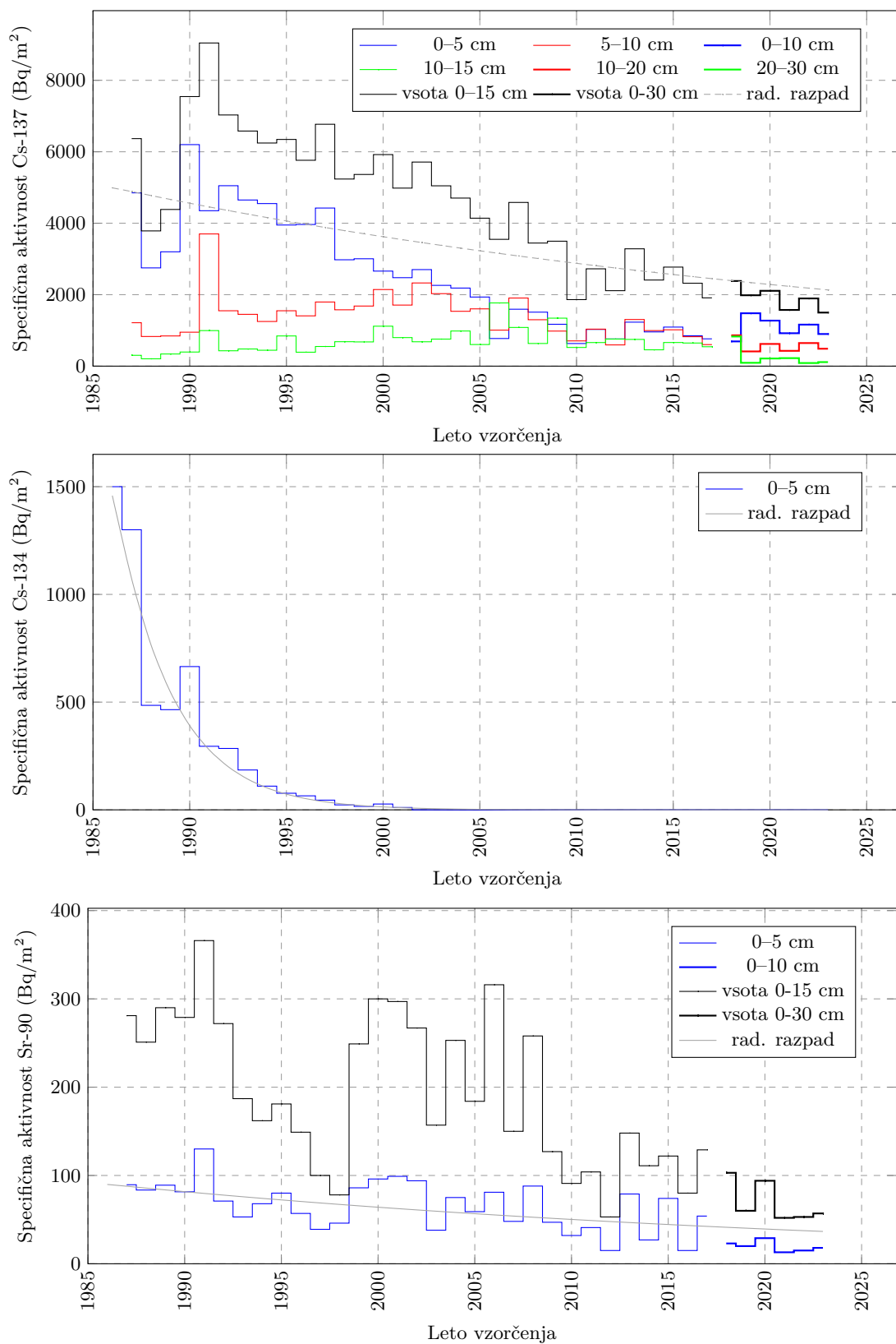
Slika 4.7 | Specifične aktivnosti — depozit — Cs-137, Cs-134 in Sr-90 v Murski Soboti v različnih plasteh ter preračun radioaktivnega razpada od leta 1986 dalje.
