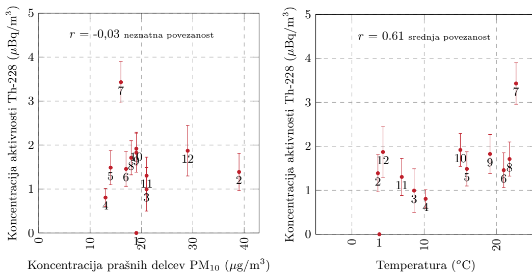
Slika 3.12 | Sezonske korelacije med aktivnostjo Th-228 v zraku in koncentracijo prašnih delcev PM 10 oziroma temperaturo v letu 2023 na lokaciji Ljubljana.
