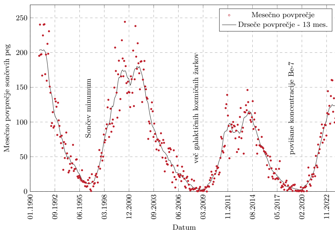
Slika 3.23 | Povprečno mesečno število sončevih peg – neprekinjena črta predstavlja drseče povprečje zadnjih 13 mesecev.
