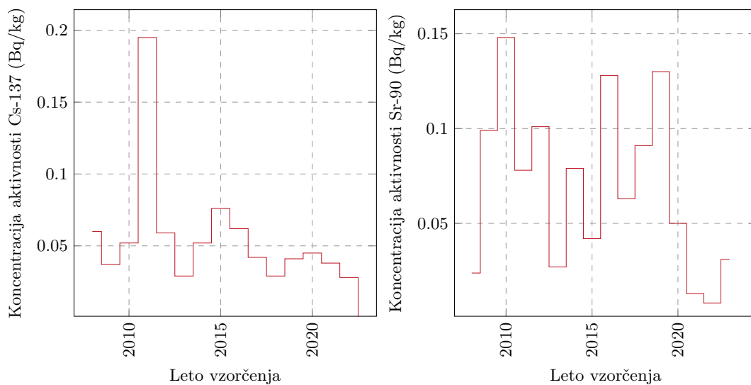
Slika 5.13 | Povprečne letne koncentracije aktivnosti Cs-137 in Sr-90 v zelenjavi od leta 2008 dalje (povprečje vseh vzetih vzorcev brez gob).
