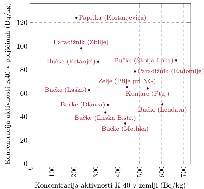
Slika 3.44 | Analiza korelacije izotopa K-40 v zemlji in poljščinah.
