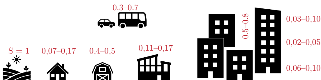
Slika 6.1 | Shematski prikaz faktorja zaradi ščitenja glede na različno vrsto zgradb.
