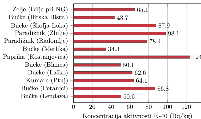
Slika 3.42 | Koncentracije K-40 v poljščinah na različnih lokacijah intenzivnega poljedelstva
