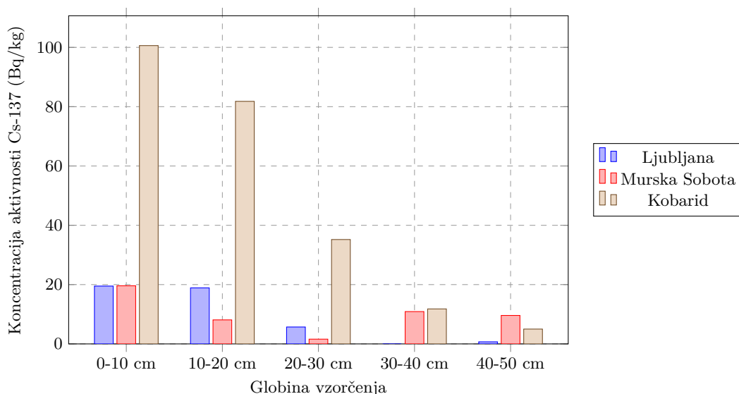
Slika 4.3 | Povprečna letna koncentracija aktivnosti Cs-137 v zemlji
