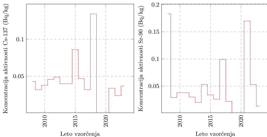
Slika 5.12 | Povprečne letne koncentracije aktivnosti Cs-137 in Sr-90 v sadju od leta 2008 dalje (povprečje vseh vzetih vzorcev razen specifičnih z večjo akumulacijo).
