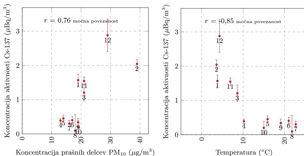
Slika 3.10 | Sezonske korelacije med aktivnostjo Cs-137 v zraku in koncentracijo prašnih delcev PM 10 oziroma temperaturo v letu 2023 na lokaciji Ljubljana.
