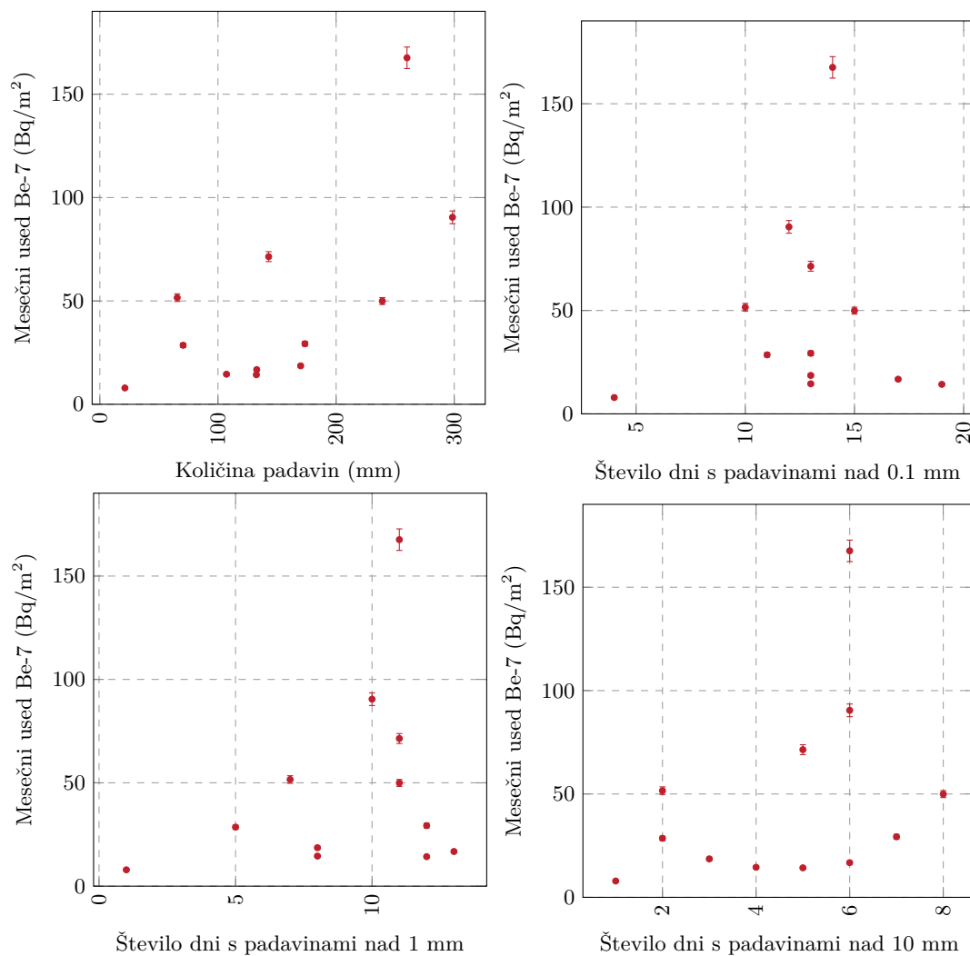
Slika 3.35 | Korelacija izmerjenega mesečnega useda Be-7 v padavinah v Ljubljani in količino padavin oziroma številom deževnih dni (za leto 2023).
