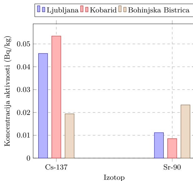
Slika 5.4 | Primerjava povprečnih letnih koncentracij aktivnosti Cs-137 in Sr-90 v surovem mleku na različnih lokacijah v Sloveniji za leto 2023.
