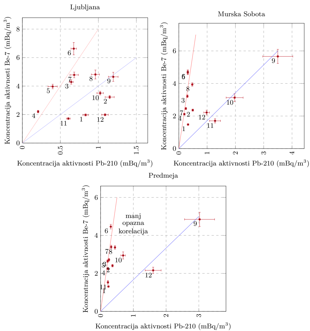
Slika 3.18 | Zimske in poletne korelacije med izmerjenimi koncentracijami atmosferskega Pb-210 in Be-7 v zraku na različnih lokacijah v letu 2023 – številka ob meritvi pomeni mesec vzorčenja.
