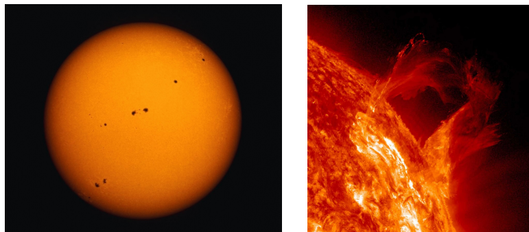
Slika 3.22 | Sončeve pege so merilo za sončevo aktivnost in solarni veter; slika: NASA.
