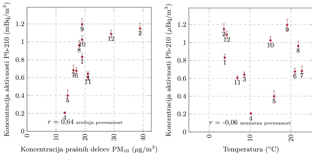
Slika 3.11 | Sezonske korelacije med aktivnostjo Pb-210 v zraku in koncentracijo prašnih delcev PM 10 oziroma temperaturo v letu 2023 na lokaciji Ljubljana.
