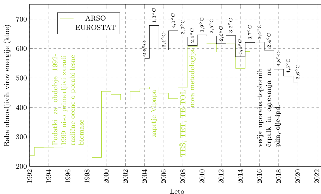
Slika 3.13 | Raba obnovljivih virov energije - les in druga trdna biomasa (ARSO) oziroma OVE za ogrevanje (EUROSTAT). Pri vsakem letu je zapisna povprečna zimsko temperatura (v času kurilne sezone – januar-februar, november-december)
