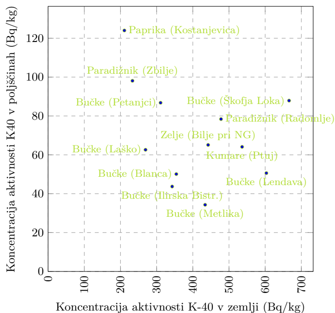
Slika 3.42 | Analiza korelacije izotopa K-40 v zemlji in poljščinah.
