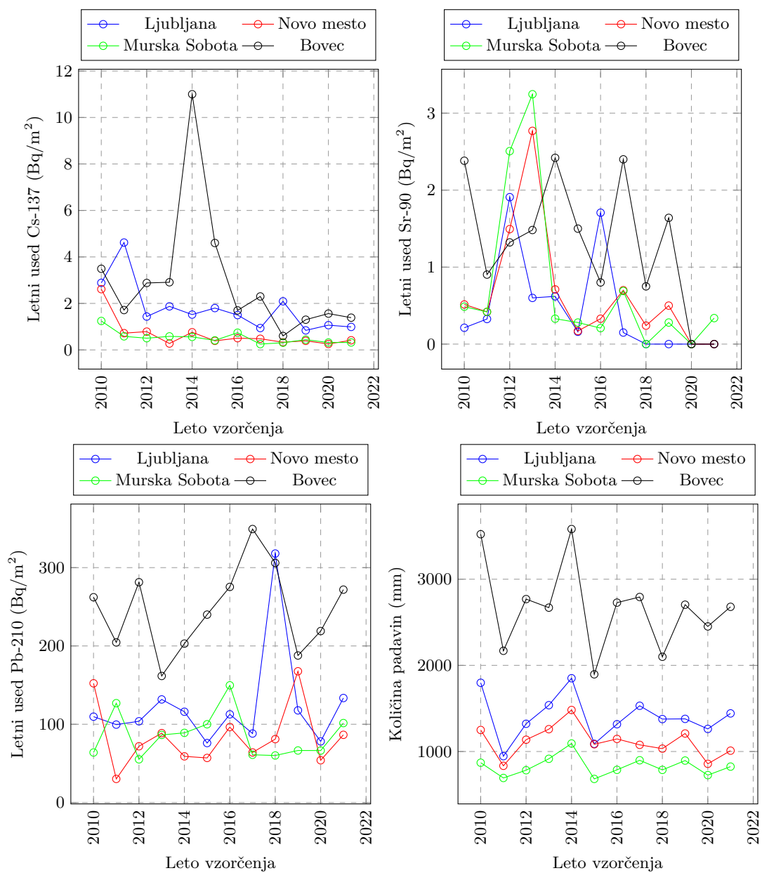
Slika 3.28 | Povprečni letni used Cs-137, Sr-90 in Pb-210 na enoto površine za obdobje od leta 2010 dalje na posamičnih lokacijah: Ljubljana, Novo mesto, Murska Sobota in Bovec.
