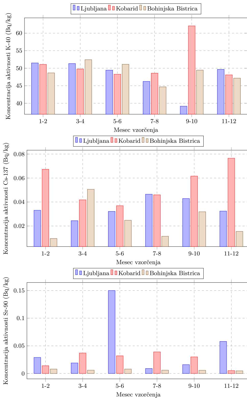
Slika 5.5 | Koncentracije aktivnosti K-40, Cs-137 in Sr-90 v posamičnih dvomesečnih vzorcih surovega mleka iz Ljubljane, Kobarida in Bohinjske Bistrice.
