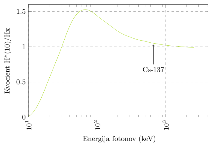
Slika 4.9 | Energijska odvisnost razmerja okoljskega, H^*(10) , in fotonskega doznega ekvivalenta, H_x .
