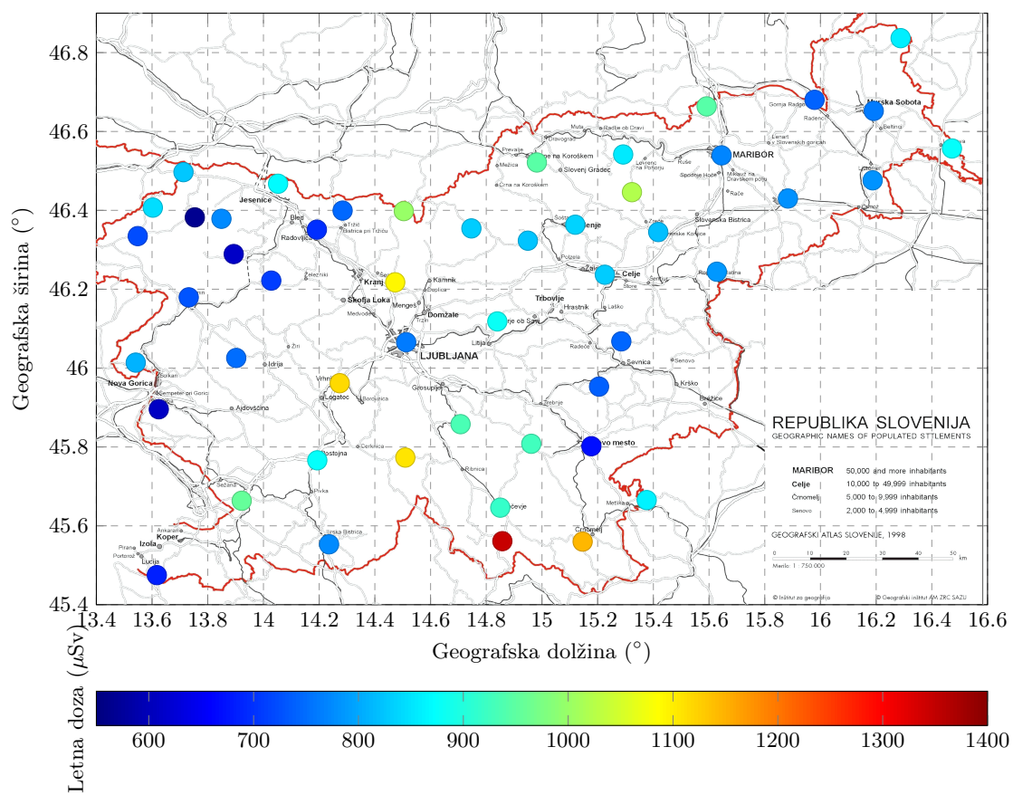
Slika 4.7 | Izmerjena letna doza s TL dozimetri na različnih lokacijah po Sloveniji.
