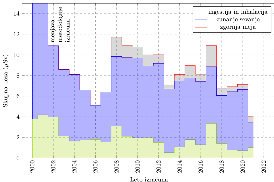
Slika 6.5 | Predvidena efektivna doza H_E zaradi kontaminacije okolja z dolgoživimi umetnimi radionuklidi za odrasle (slovensko povprečje) za obdobje od leta 2000 dalje
