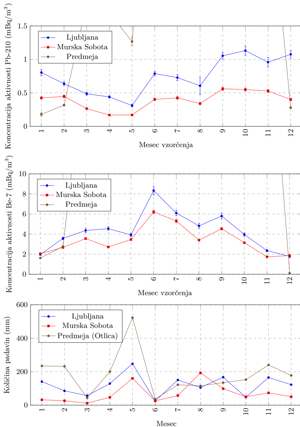
Slika 3.16 | Sezonska variacija koncentracij atmosferskega Pb-210 in Be-7 v zraku in padavin na bližnjih lokacijah.
