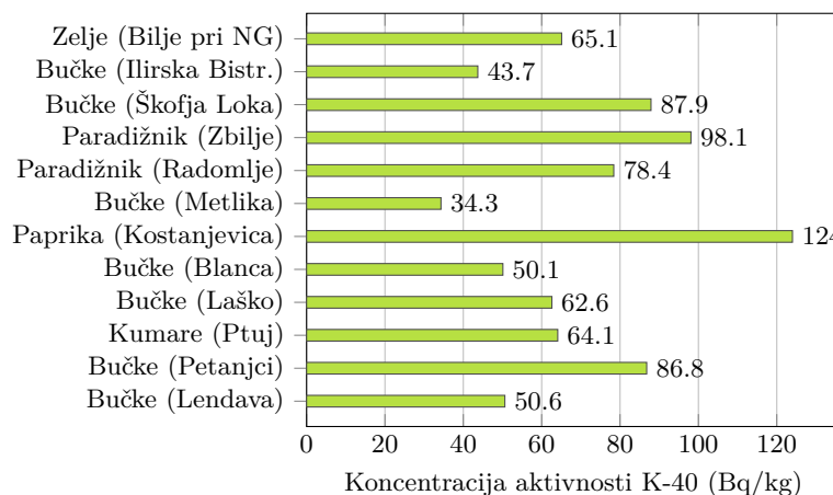
Slika 3.40 | Koncentracije K-40 v poljščinah na različnih lokacijah intenzivnega poljedelstva
