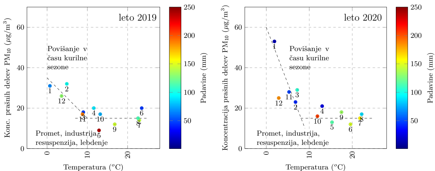
Slika 3.10 | Zgodovinski pregled temperaturne korelacije prašnih delcev PM_{10} na lokaciji v Ljubljani - nadaljevanje.
