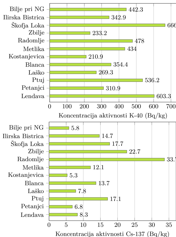
Slika 3.38 | Koncentracije K-40 in Cs-137 v obdelani zemlji na poljedeljsko intenzivnih območjih
