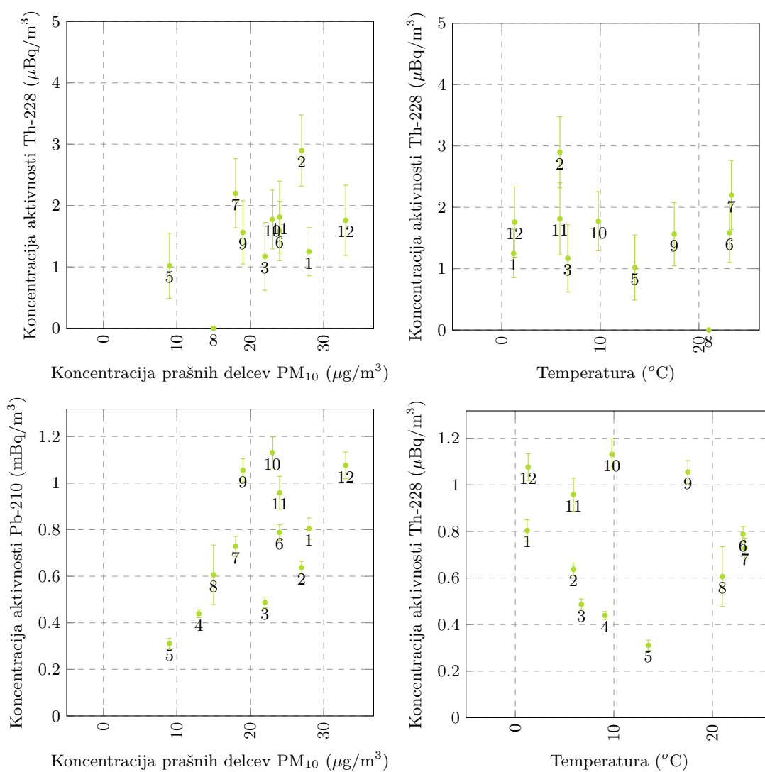
Slika 3.12 | Sezonske korelacije med aktivnostjo naravnih radionuklidov, Th-228 in Pb-210, v zraku in koncentracijo prašnih delcev PM 10 oziroma temperaturo na lokaciji Ljubljana.
