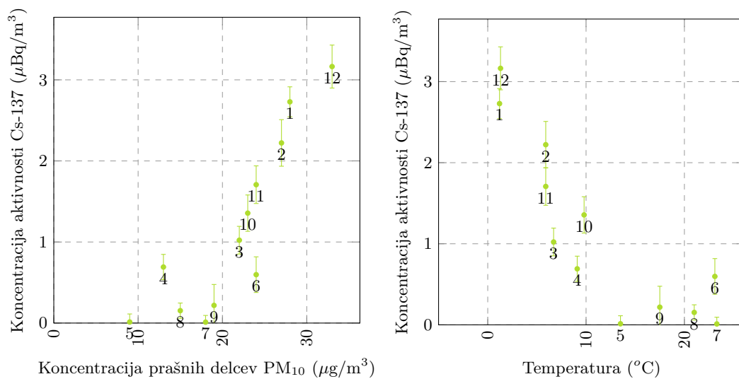
Slika 3.11 | Sezonske korelacije med aktivnostjo Cs-137 v zraku in koncentracijo prašnih delcev PM_{10} oziroma temperaturo na lokaciji Ljubljana.
