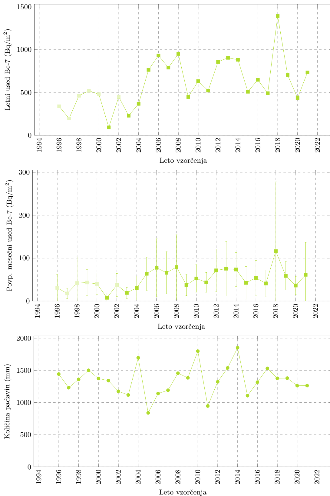
Slika 3.31 | Specifične aktivnosti Be-7 v padavinah iz Ljubljane za obdobje od leta 1996 dalje.
