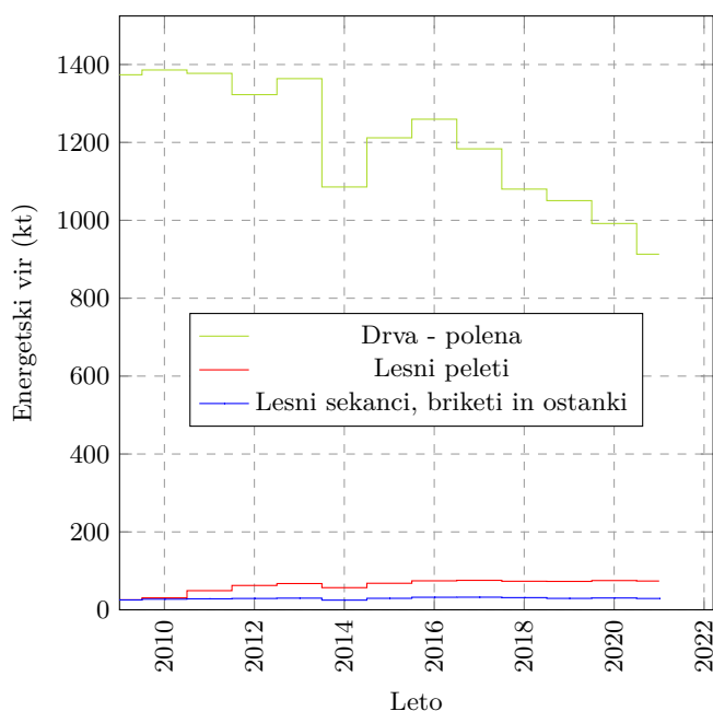
Slika 3.14 | Končna poraba energije lesnih kuriv v gospodinjstvih izračunana s pomočjo modela rabe energije v gospodinjstvih (IJS-CEU). Vrednosti za leto 2021 so ocenjene z linearno ekstrapolacijo trenda preteklih 5 let.
