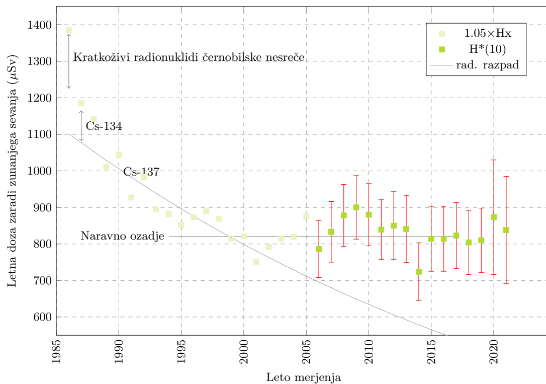
Slika 4.8 | Doza zaradi zunanega sevanja za Ljubljano za obdobje od leta 1986 dalje.
