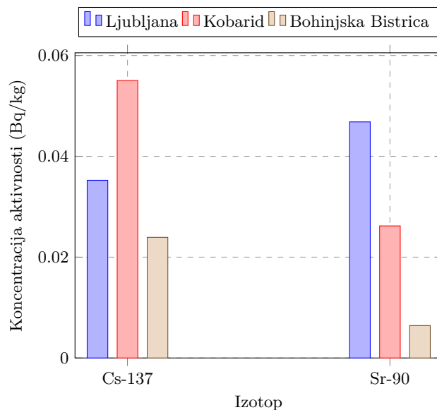
Slika 5.4 | Primerjava povprečnih letnih koncentracij aktivnosti Cs-137 in Sr-90 v surovem mleku na različnih lokacijah v Sloveniji za leto 2021.
