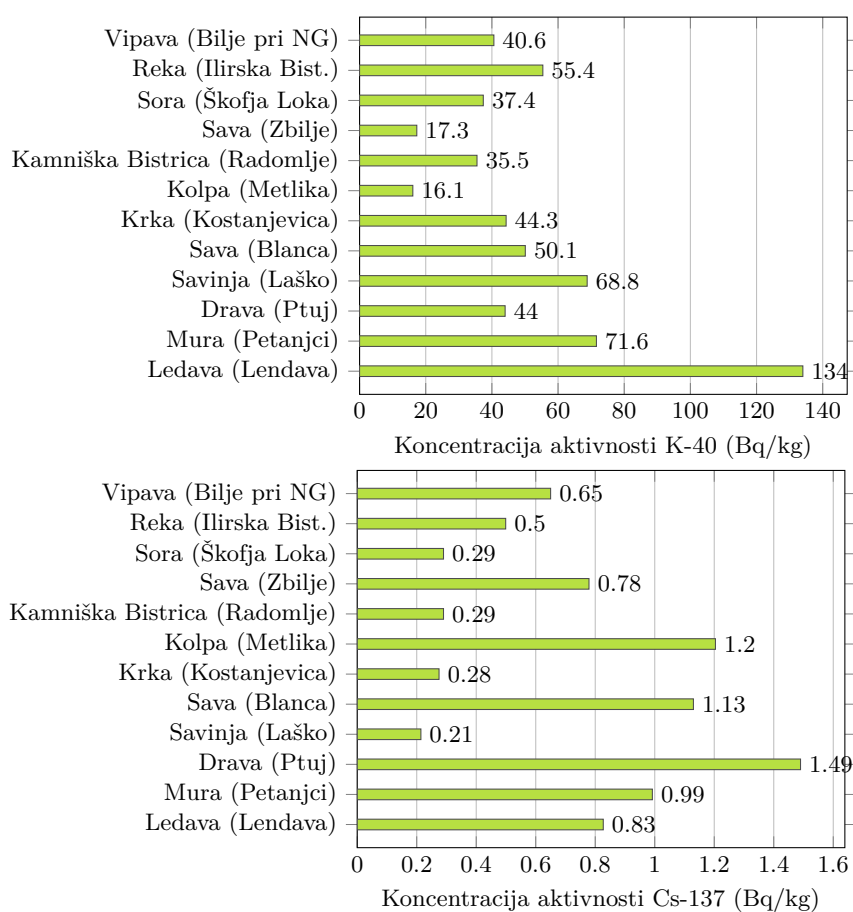
Slika 3.39 | Koncentracije K-40 in Cs-137 v nefiltrirani rečni vodi na različnih lokacijah intenzivnega poljedelstva
