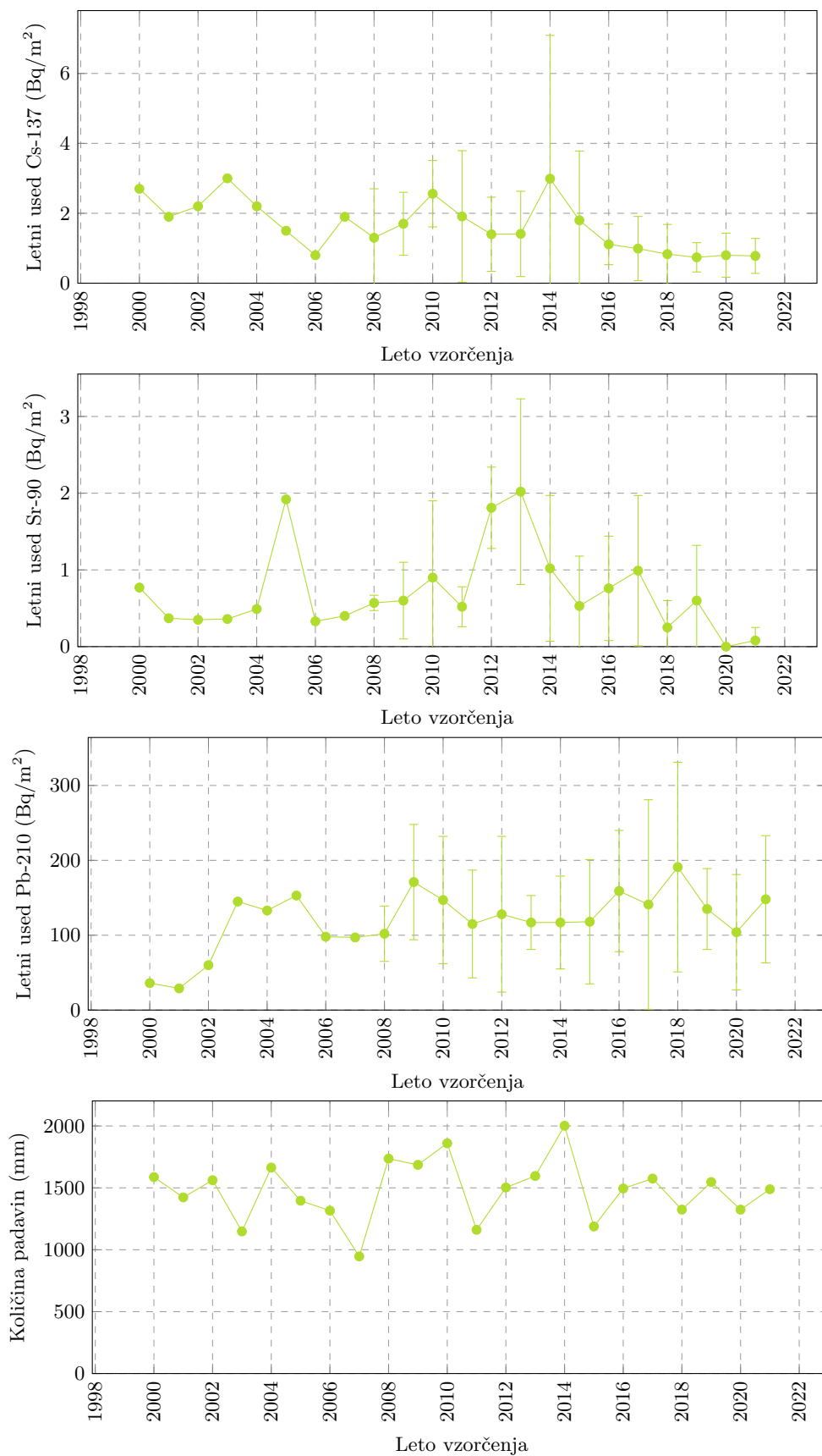
Slika 3.27 | Povprečni letni used Cs-137, Sr-90 in Pb-210 na enoto površine za obdobje od leta 2000 dalje (povprečje vseh lokacij po Sloveniji)
