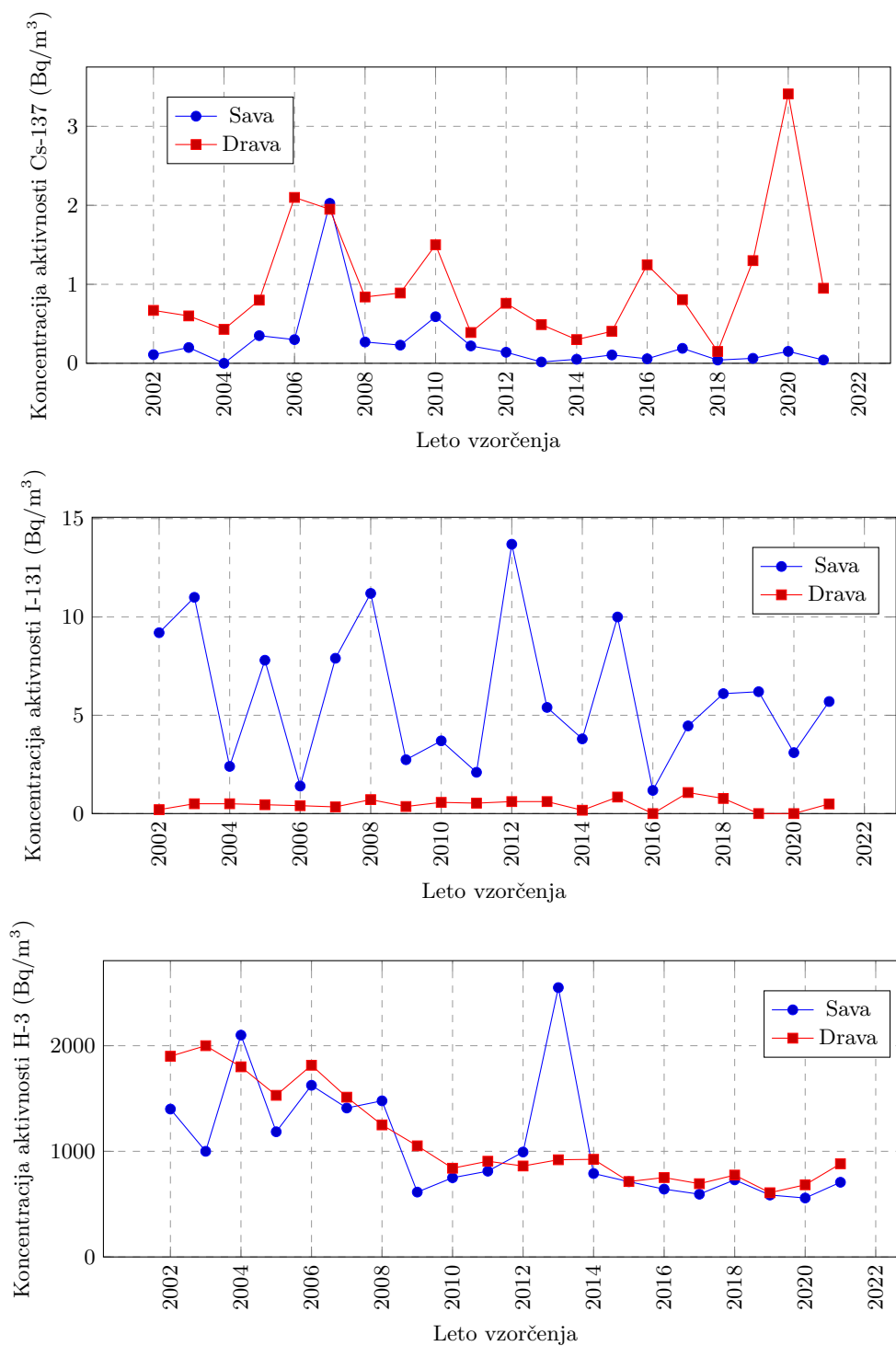
Slika 3.36 | Povprečne letne koncentracije aktivnosti Cs-137, I-131 in H-3 v reki Savi (povprečje lokacij Ljubljana in Brežice) in Dravi od leta 2002 dalje.
