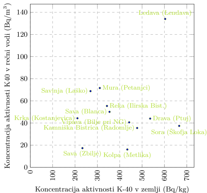
Slika 3.41 | Analiza korelacije izotopa K-40 v obdelani zemlji in nefiltrirani rečni vodi.
