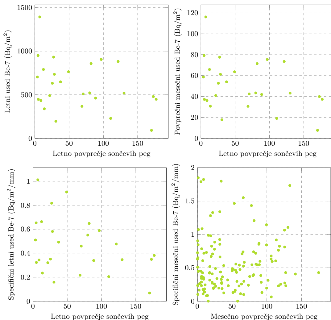
Slika 3.32 | Korelacija skupnega letnega useda, povprečnega mesečnega useda in specifičnega letnega ter specifičnega mesečnega useda Be-7 s sončevim ciklom od leta 1996 dalje.
