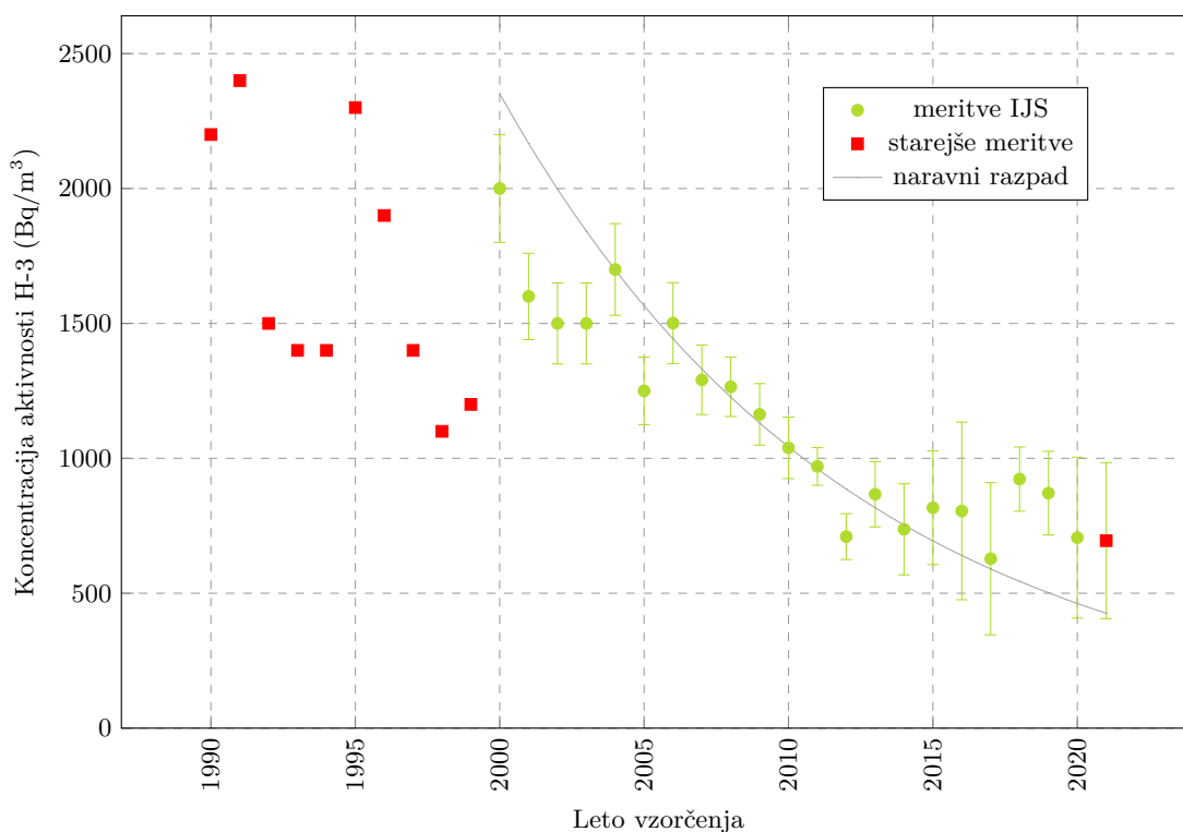
Slika 3.30 | Povprečne letne koncentracije aktivnosti H-3 v padavinah iz Ljubljane za obdobje od leta 1990 dalje.
