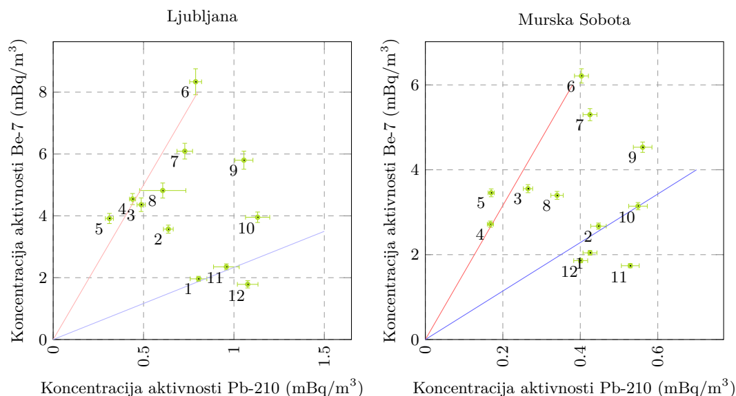
Slika 3.18 | Zimske in poletne korelacije med izmerjenimi koncentracijami atmosferskega Pb-210 in Be-7 v zraku na različnih lokacijah v letu 2021 – številka ob meritvi pomeni mesec vzorčenja.
