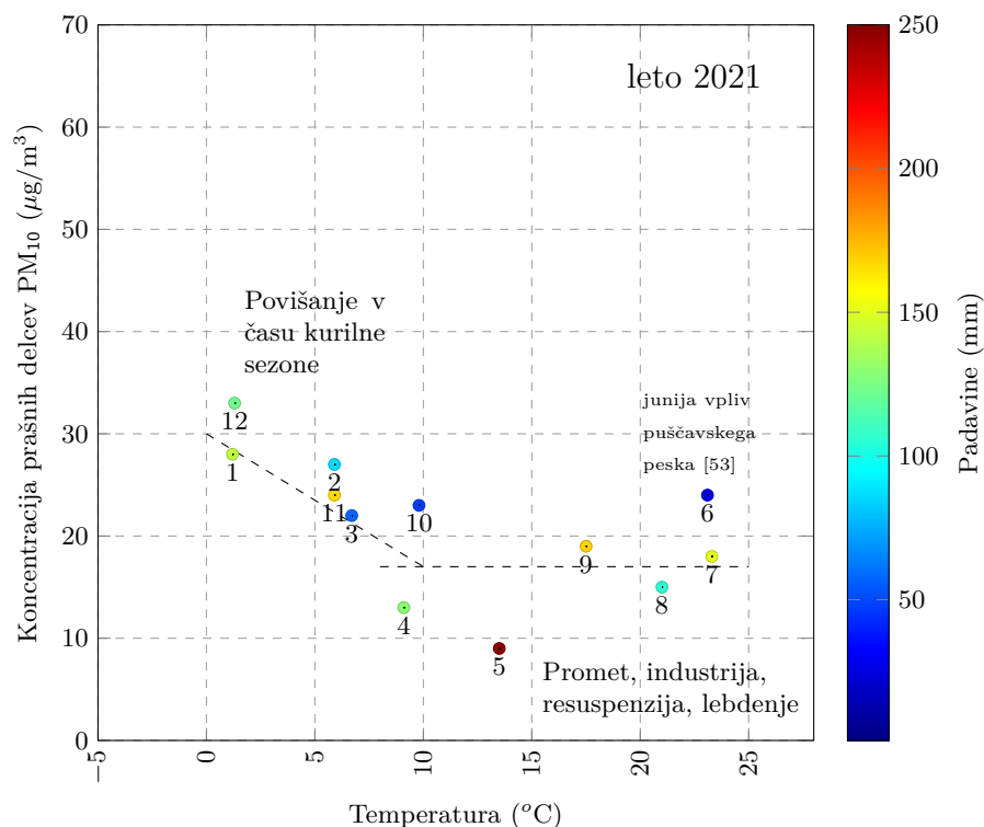
Slika 3.8 | Temperaturna korelacija prašnih delcev PM_{10} za preteklo leto na lokaciji v Ljubljani – oznake ob merskih točkah predstavljajo mesec meritve, barvna oznaka pa količino padavin.
