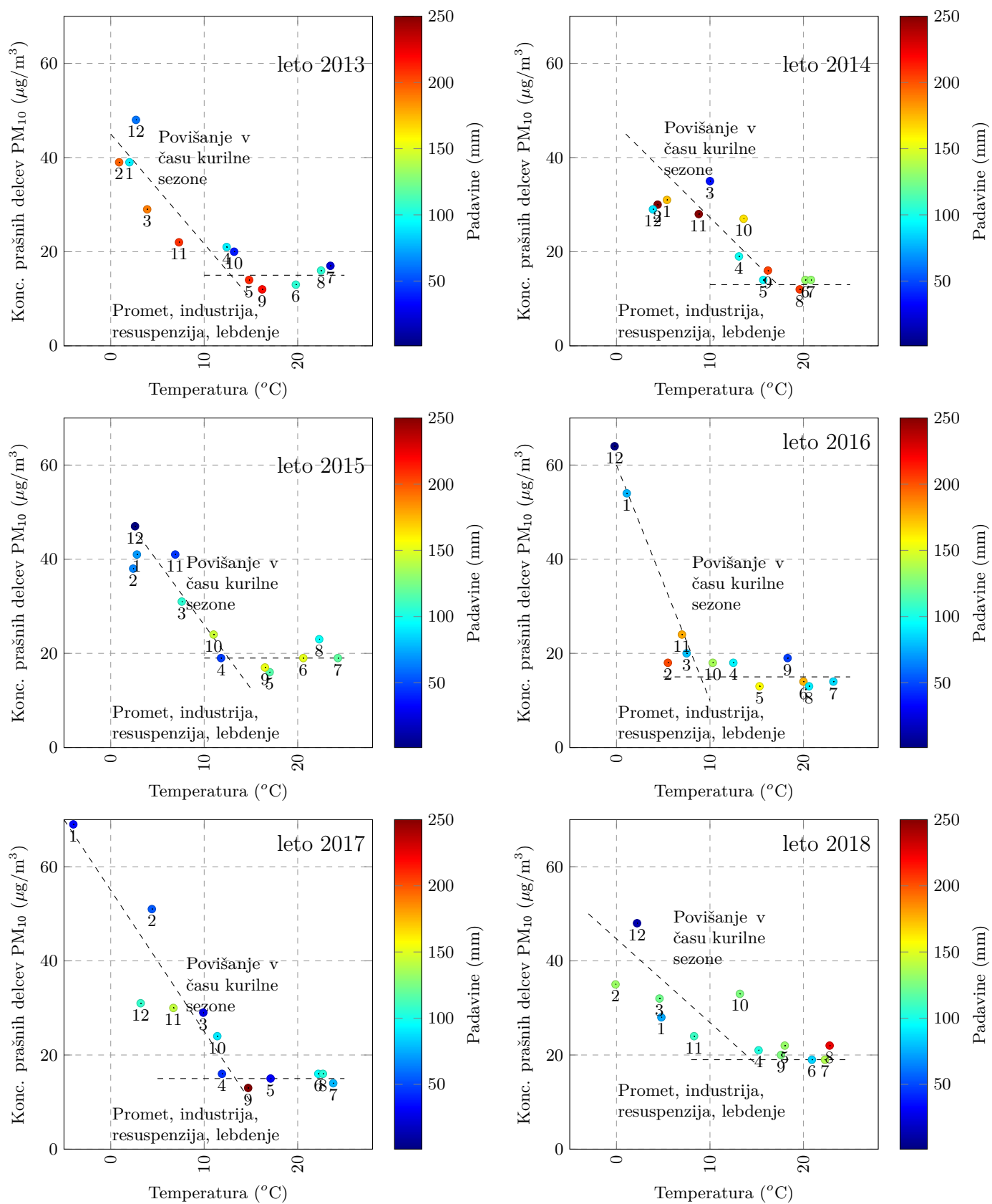
Slika 3.9 | Zgodovinski pregled temperaturne korelacije prašnih delcev \text{PM}_{10} na lokaciji v Ljubljani.
