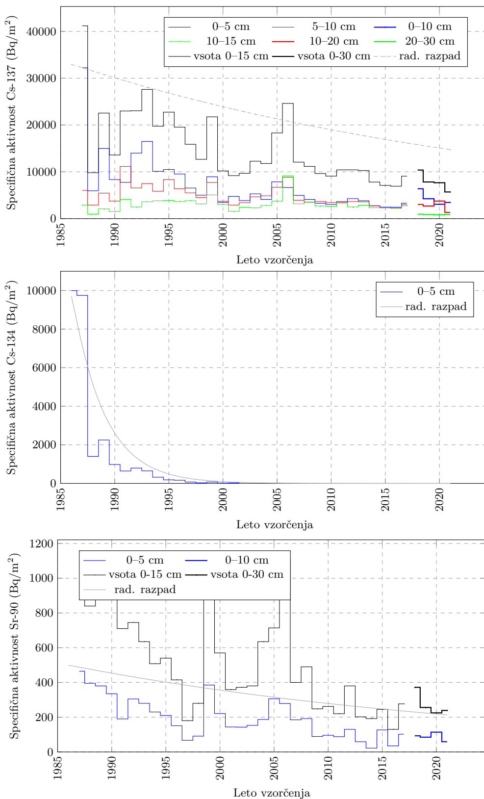
Slika 4.4 | Specifične aktivnosti — deposit — Cs-137, Cs-134 in Sr-90 v Kobaridu v različnih plasteh ter preračun radioaktivnega razpada od leta 1986 dalje.
