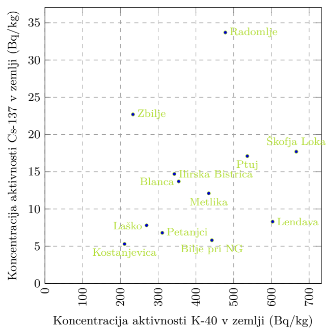
Slika 3.43 | Analiza korelacije izotopa K-40 in Cs-137 v zemlji.
