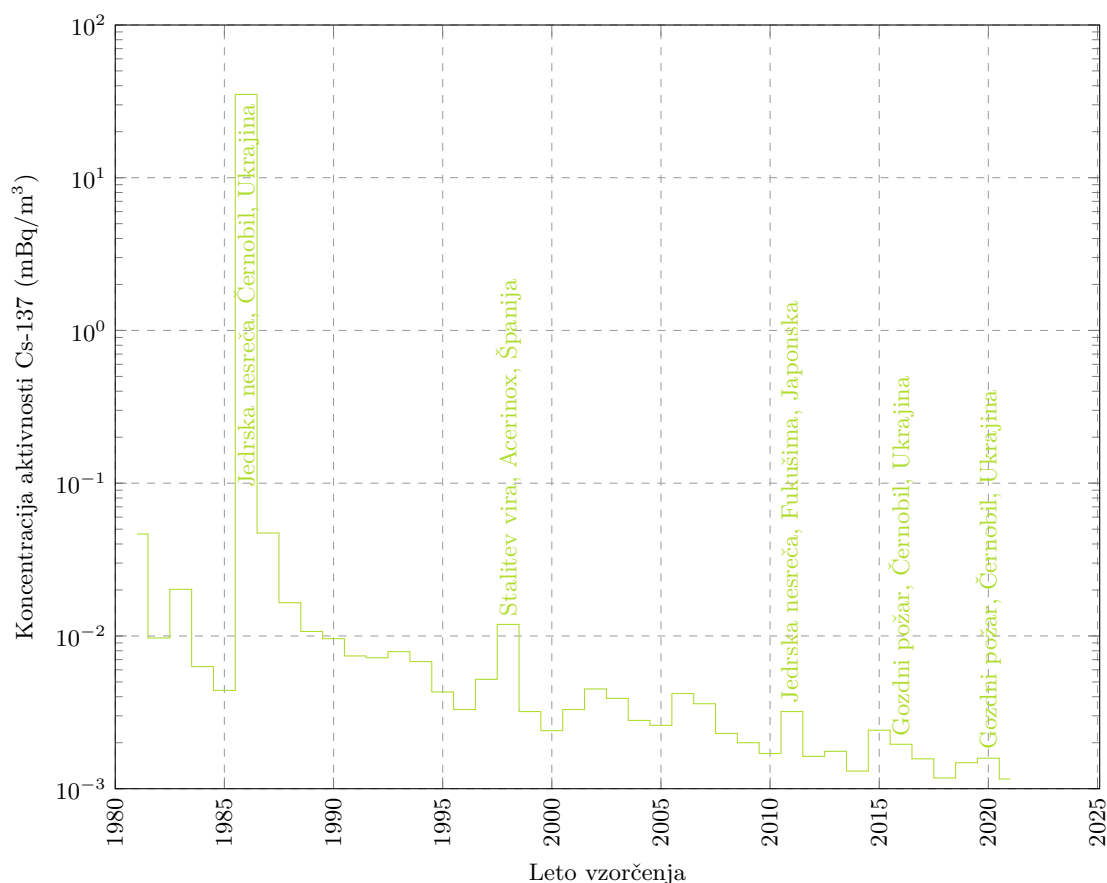
Slika 3.2 | Letna povprečja koncentracij aktivnosti Cs-137 v zraku na lokaciji Ljubljana od leta 1981 dalje
