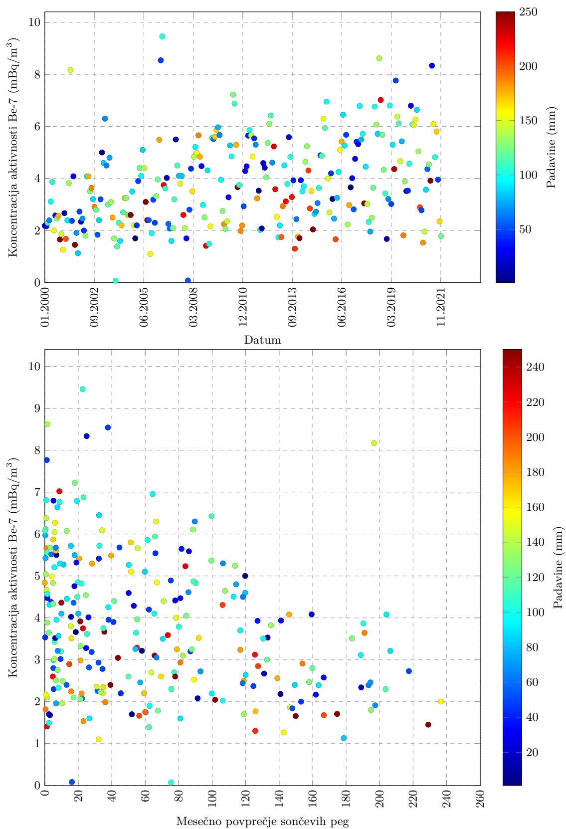
Slika 3.25 | Antikorelacija sončevega cikla z mesečnimi koncentracijami Be-7 v zraku od leta 2000 dalje z delnim upoštevanjem izpiranja zaradi padavin.
