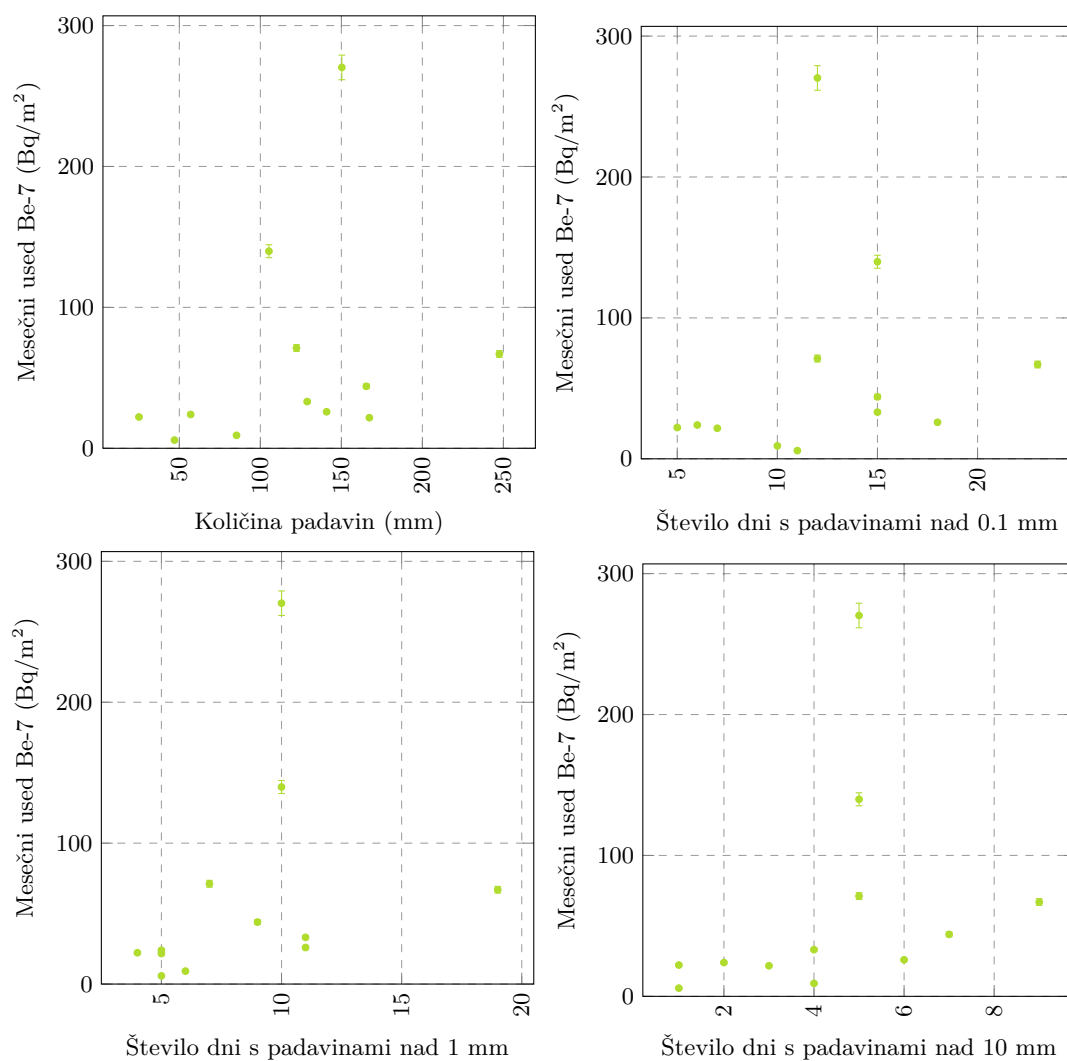
Slika 3.33 | Korelacija izmerjenega mesečnega usoda Be-7 v padavinah v Ljubljani in količino padavin oziroma številom deževnih dni (za leto 2021).
