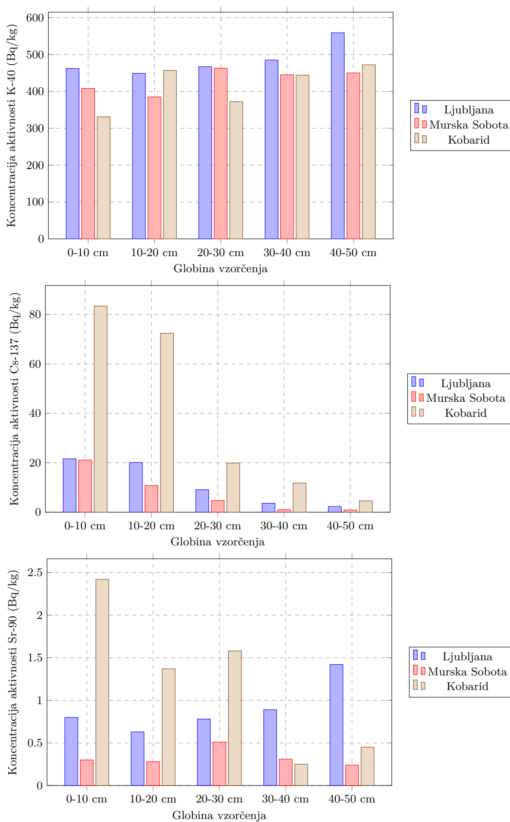
Slika 4.2 | Povprečna letna koncentracija aktivnosti K-40, Cs-137 in Sr-90 v zemlji
