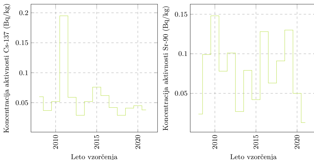
Slika 5.11 | Povprečne letne koncentracije aktivnosti Cs-137 in Sr-90 v zelenjavi od leta 2008 dalje (povprečje vseh vzorčev brez gob).
